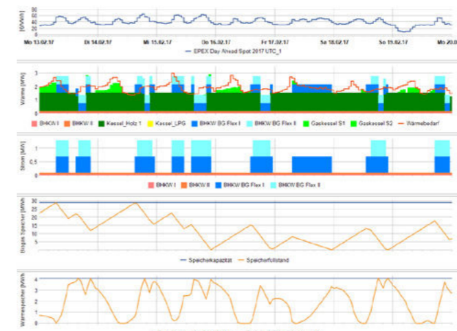
Abb. 2: Simulation des flexiblen BHKW-Betriebs
