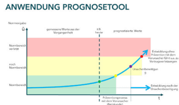
Abbildung 1: Anwendungsbeispiel Frühwarnsystem für Oberschwingungen
