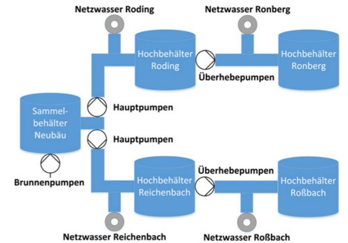
Abbildung 2: Schematischer Aufbau des Pumpenmodells
