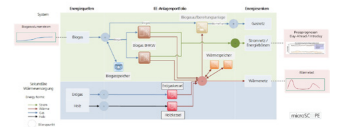
Abb. 3: Anlagenmodell für die Betriebsoptimierung
