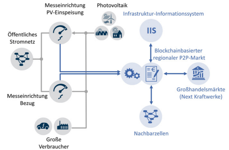
Abbildung 1: Einbindung des lokalen Marktes in das zelluläre Energiesystem.
